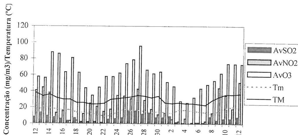
Fig. 3 – Comparação entre a variação da concentração dos poluentes e a temperatura em Teixugueira (período de 12 de Junho a 12 de Julho de 1996 – \text{mg/m}^3 e ^{\circ}\text{C} )
