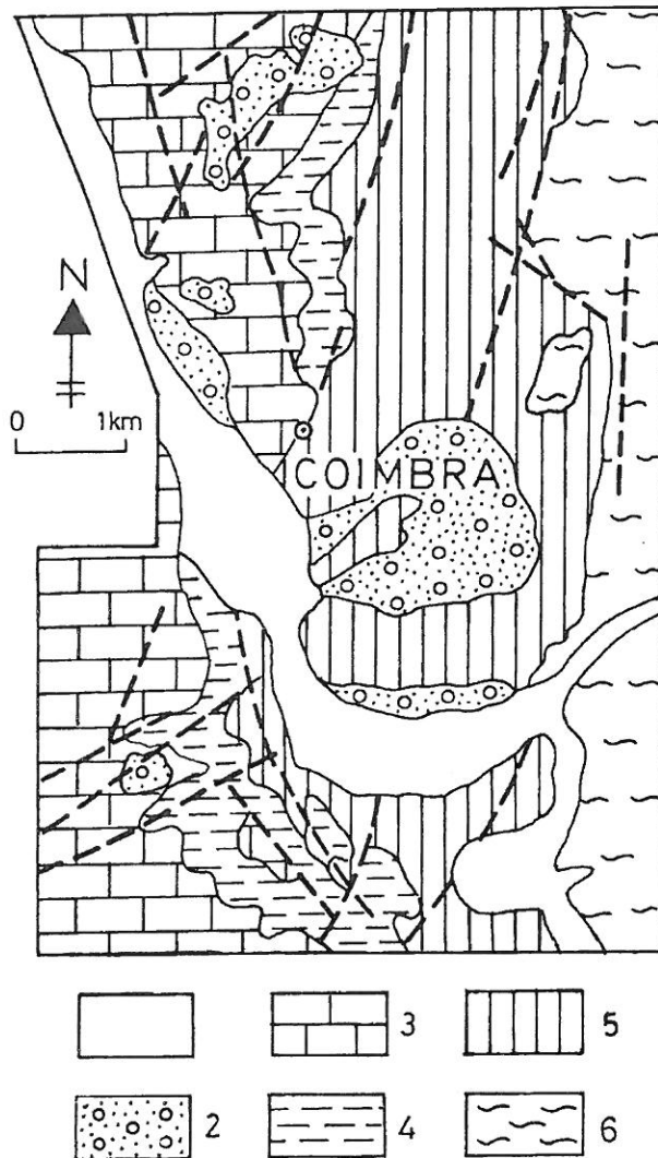
Fig. 1 - Mapa geológico simplificado da região de Coimbra. Símbolos: 1 - aluvião; 2 - rochas detriticas quaternárias; 3 - rochas carbonatadas do jurássico médio; 4 - rochas do jurássico inferior, com componente carbonatada e detritica; 5 - rochas detriticas triásicas; 6 - rochas metassedimentares precâmblicas; falhas a tracejado grosso.
