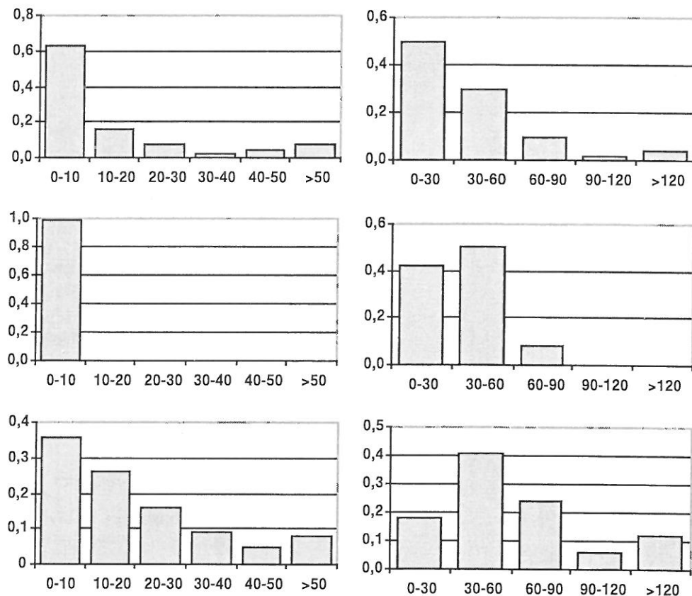
Fig. 2 – Histogramas da distribuição das concentrações de radão medidas nos solos da região de Coimbra, à esquerda (expressas em \text{kBq.m}^{-3} ), e em habitações da mesma região, à direita (expressas em \text{Bq.m}^{-3} ); as ordenadas são frequências relativas. De cima para baixo estão sucessivamente representados os dados referentes a substrato de rochas detríticas triásico-hetangianas, de rochas carbonatadas jurássicas e de rochas detríticas quaternárias. (Segundo NEVES et al. , 1999).
