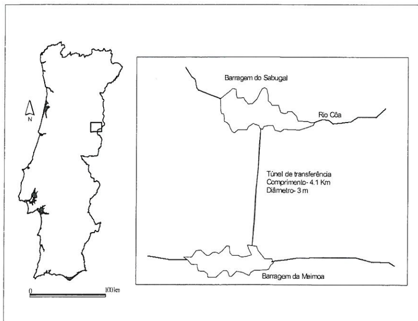
Figura 2 Localização do circuito hidráulico composto pelas barragens do Sabugal/Meimosa
