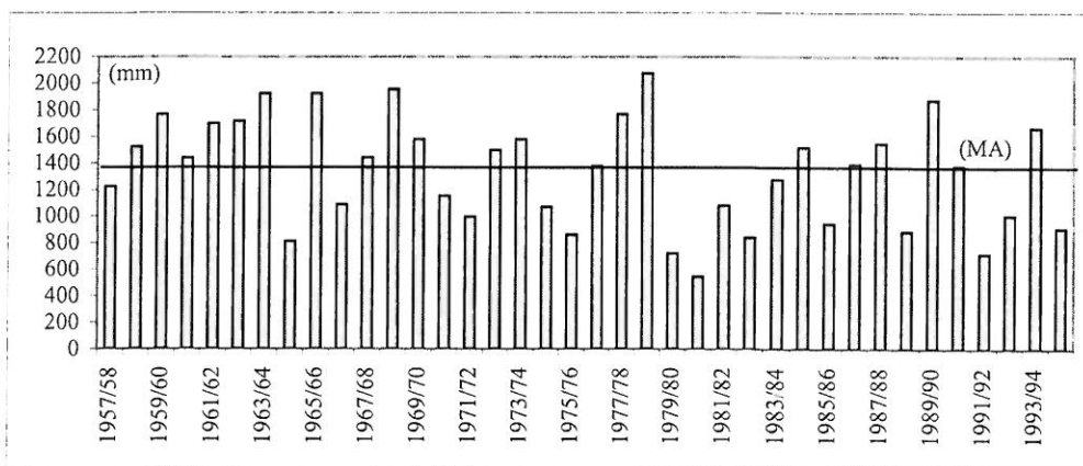
Figura 3 Precipitação total anual e valor médio anual (MA) no Posto de Vale de Espinho (Fonte: INAG)
