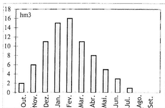
Figura 4 Escoamentos médios na secção da barragem do Sabugal em hm³ (1960-90). (Fonte: ESTUDO DE IMPACTE AMBIENTAL, 1994)
