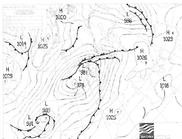
Figura 1 Carta sinóptica de 25/10/05 ( http://www.infomet.fcr.es/ )
