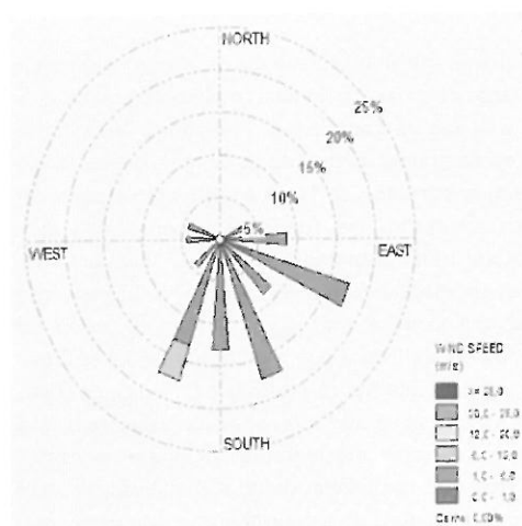
Gráfico 1 Rosa anemoscópica respeitante a 25/10/05 (elaboração própria)
