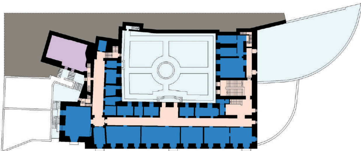
Piso 1A Floor 1A
