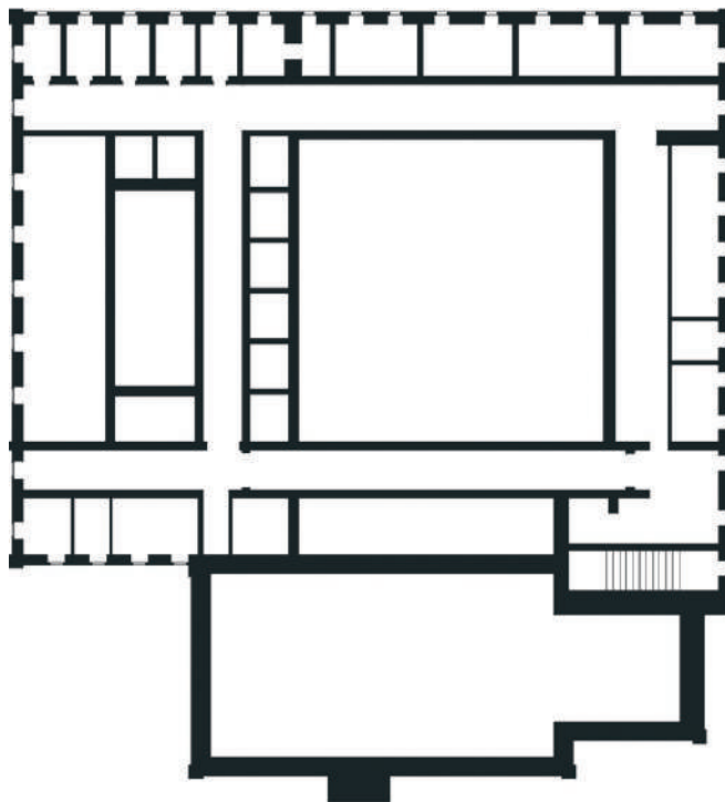
Piso 2A Floor 2A
