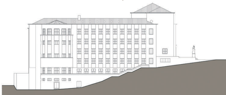
Corte poente — nascente pelo pátio West-East cross section of the courtyard
