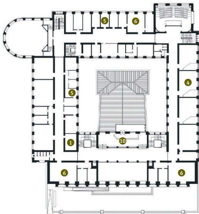
Piso 3A Floor 3A
