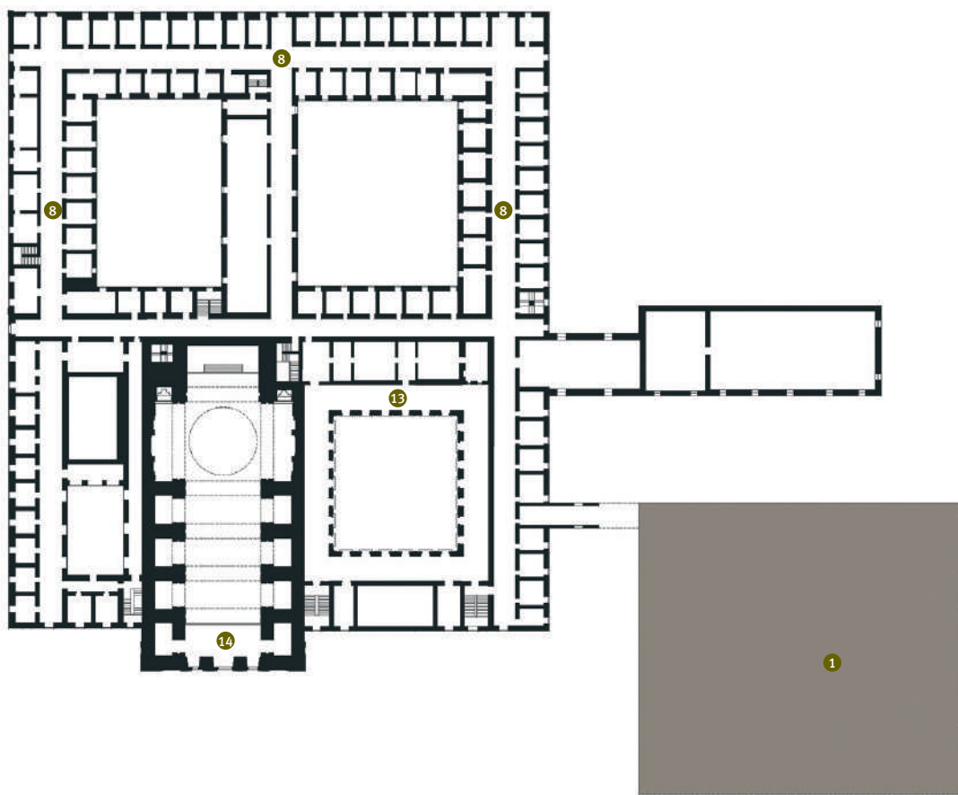
Piso 1A Floor 1A
